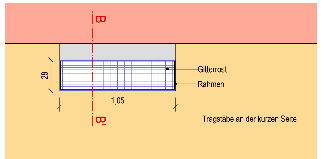
GRUNDRISS LICHTSCHACHTABDECKUNG
